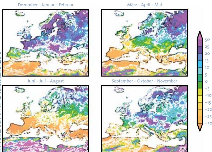
Prognose der Niederschlagsveränderungen (%) für den Zeitraum von 2071 bis 2100, bezogen auf die mittleren Niederschläge von 1961 bis 1990
